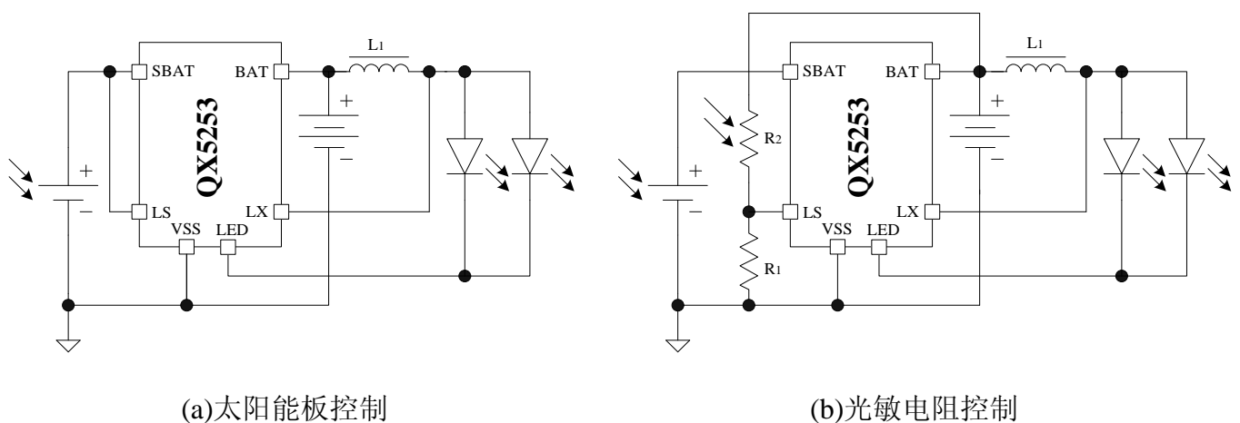
图 1: QX5253 典型应用电路图
