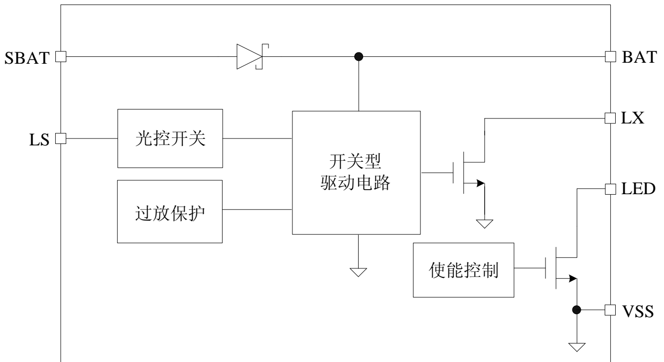
图 2: QX5253 的内部电路方框图
